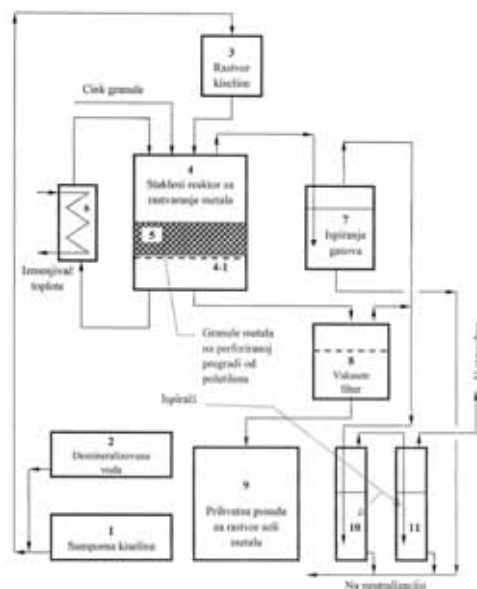
Sl.1. Shema postrojenja za rastvaranje metala u kiselinama, odnosa, cinka u rastvoru sumporne kiseline
