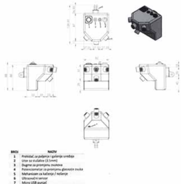
Slika 3. Prototip
